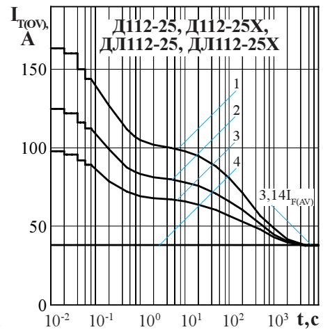
Рисунок 10 - Зависимость допустимой амплитуды прямого тока перегрузки I_{T(OV)} синусоидальной формы частотой f = 50 Гц от длительности перегрузки t при температуре окружающей среды T_a = 40 °С и при отношении тока, предшествующего перегрузке, I_F к допустимому среднему прямому току с охладителем I_{F(AV)} равному k = I_F / I_{F(AV)} ; k = 0 (1); 0,5 (2); 0,75 (3); 1,0 (4).
