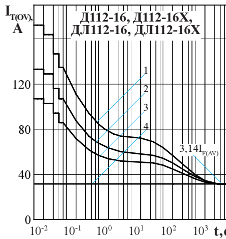
Рисунок 10 - Зависимость допустимой амплитуды прямого тока перегрузки I_{T(OV)} синусоидальной формы частотой f = 50 Гц от длительности перегрузки t при температуре окружающей среды T_a = 40 °С и при отношении тока, предшествующего перегрузке, I_F к допустимому среднему прямому току с охладителем I_{F(AV)} равному k = I_F / I_{F(AV)} ; k = 0 (1); 0,5 (2); 0,75 (3); 1,0 (4).
