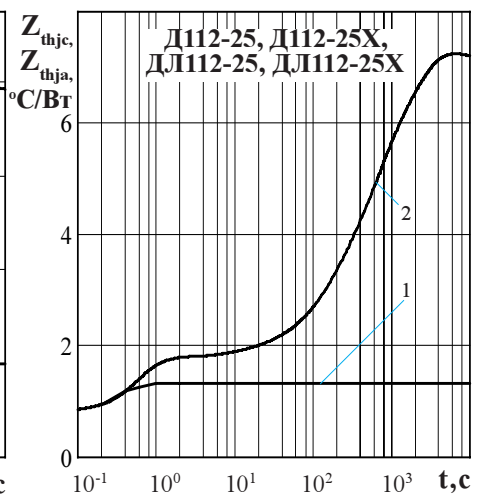
Рисунок 11 - Зависимость теплового сопротивления переход - корпус Z_{thjc} (1) и переход- среда Z_{thja} (2) от времени t при естественном охлаждении T_a = 40 °С на типовом охладителе.
