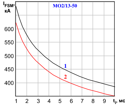
Рисунок 3: Зависимость допустимой амплитуды ударного прямого тока диодного элемента , входящего в состав модуля, I_{FSM} от длительности импульса тока t_i при исходной температуре структуры T_j=25^\circ\text{C} (1) и максимально допустимой температуре перехода T_{jm} (2).
