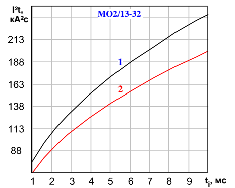
Рисунок 4: Зависимость защитного показателя диодного элемента , входящего в состав модуля, I^2t от длительности импульса тока t_i при исходной температуре структуры T_j=25^\circ\text{C} (1) и максимально допустимой температуре перехода T_{jm} (2).
