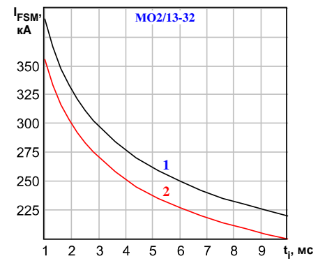
Рисунок 3: Зависимость допустимой амплитуды ударного прямого тока диодного элемента , входящего в состав модуля, I_{FSM} от длительности импульса тока t_i при исходной температуре структуры T_j=25^\circ\text{C} (1) и максимально допустимой температуре перехода T_{jm} (2).
