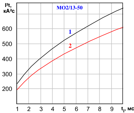
Рисунок 4: Зависимость защитного показателя диодного элемента , входящего в состав модуля, I^2t от длительности импульса тока t_i при исходной температуре структуры T_j=25^\circ\text{C} (1) и максимально допустимой температуре перехода T_{jm} (2).
