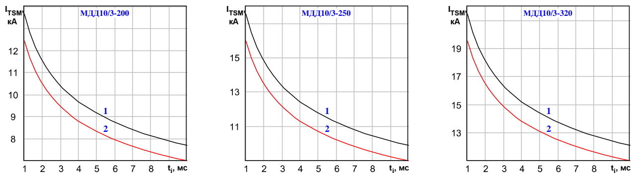
Рисунок 4: Зависимость допустимой амплитуды ударного прямого тока I_{TSM} от длительности импульса тока t_i при исходной температуре структуры T_j=25\text{ }^\circ\text{C} (1) и максимально допустимой температуре перехода T_{jm} (2).
