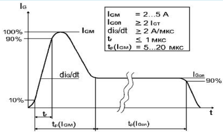
Рисунок 16: Рекомендуемая форма импульса управления. t(I_{Gon}) - определяется характеристиками тиристора и режимом работы преобразователя.
