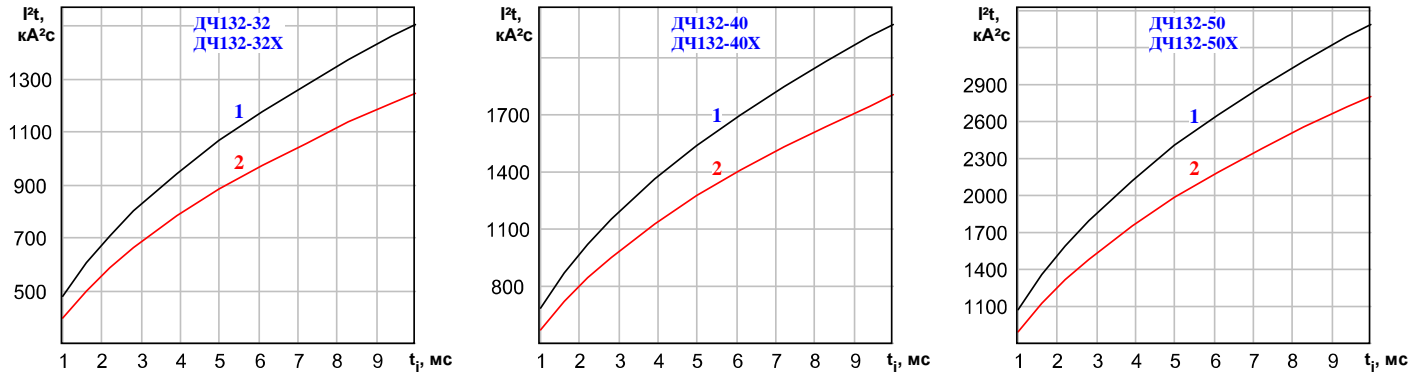
Рисунок 5: Зависимость защитного показателя I^2t от длительности импульса тока t_p при исходной температуре структуры T_j=25^\circ\text{C} (1) и максимально допустимой температуре перехода T_{jm} (2).
