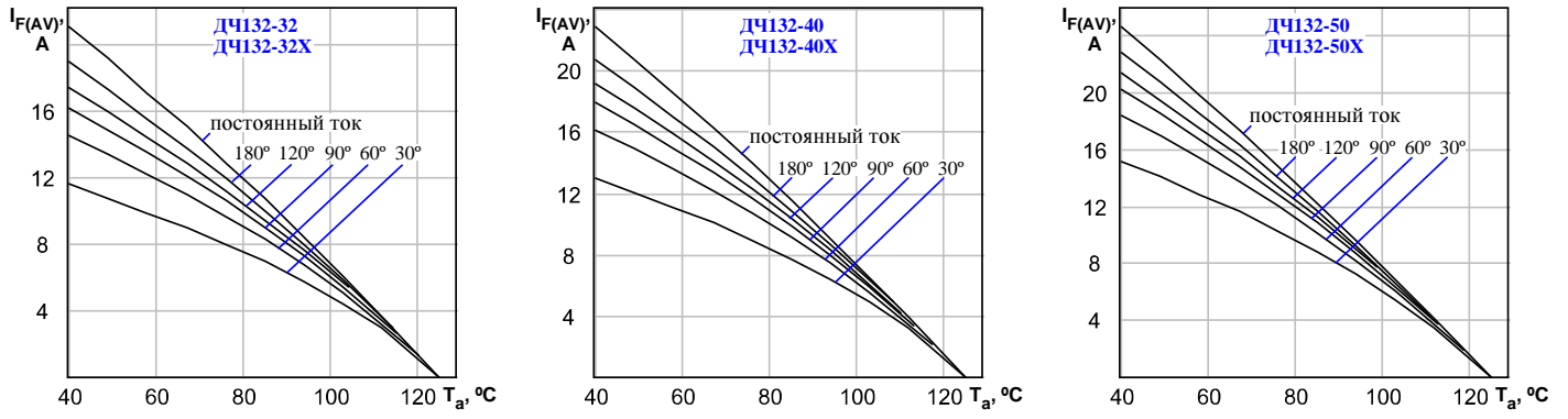
Рисунок 9: Зависимость допустимого среднего прямого тока I_{F(AV)} прямоугольной формы частотой 50 Гц при различных углах проводимости и постоянного тока от температуры окружающей среды T_a при естественном охлаждении на ОР331-80.
