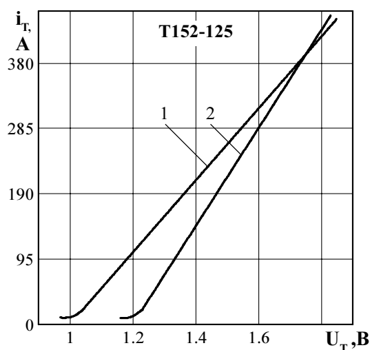
Рисунок 1 - Пределная вольтамперная характеристика в открытом состоянии при температуре перехода 25\text{ }^\circ\text{C} (1) и максимальной температуре перехода T_{jm} (2) I_T = 3,14I_{T(AV)}
